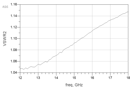
功分口驻波
