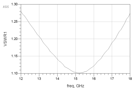
合成口驻波
