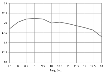
小信号增益
