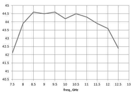
饱和输出功率, Pin=27dBm
