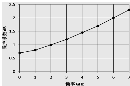
噪声系数
