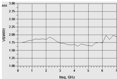
输入驻波
