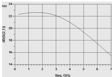
小信号增益
