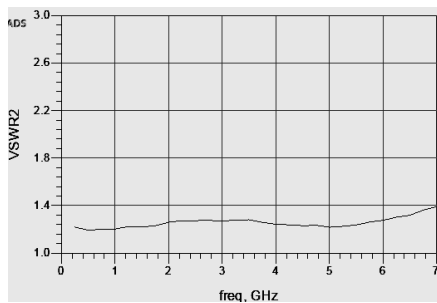
输出驻波
